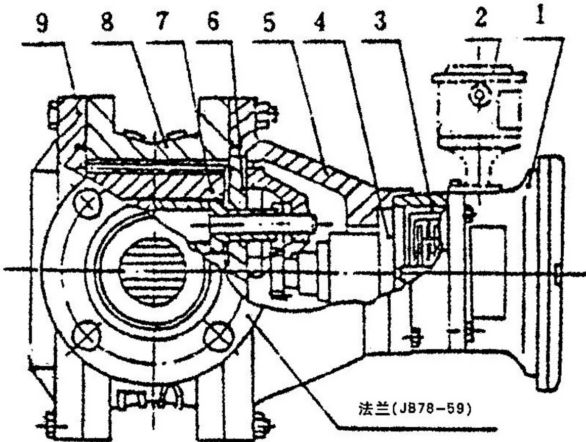
(图2) 椭圆齿轮流量计结构图
